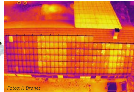
Die Hochleistungswärmebildkamera kommt bei der Thermografie zum Einsatz z.B. bei der Inspektion von PV-Anlagen.
